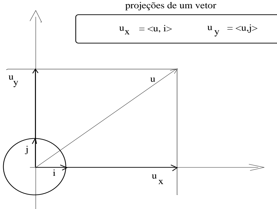
Figura 1: produto escalar e projeções de um vetor
